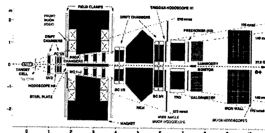
Рис. 1: Спектрометр HERMES.
