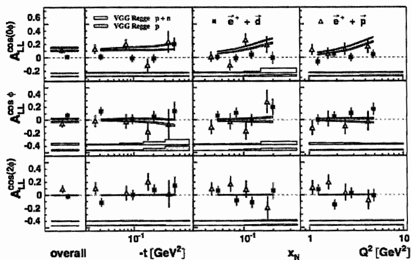
Рис. 9: Амплитуды асимметрии A_{LL} на протоне и дейтроне.
