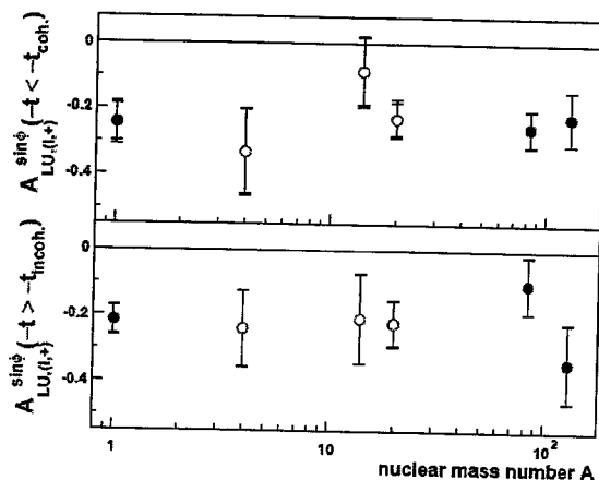
Рис. 12: А-зависимость \sin\phi амплитуды асимметрии A_{LU(l,+)} для когерентно-обогащенной и некогерентно-обогащенной областей.
