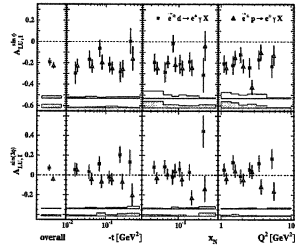
Рис. 6: Амплитуды асимметрии A_{LU,I} на неполяризованном дейтроне и протоне.
