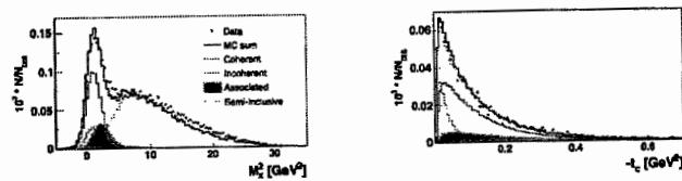
Рис. 2: Распределения недостающей массы и четырехмерного переданного импульса.
