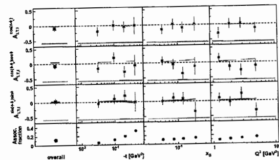
Рис. 11: Амплитуды усредненной по заряду двойной-спиновой асимметрии.
