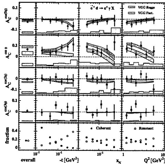
Рис. 3: Амплитуды зарядовой асимметрии на неполяризованном дейтроне.
