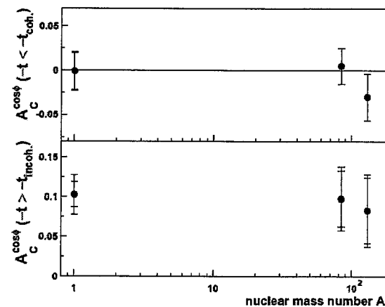
Рис. 13: А-зависимость \cos\phi амплитуды асимметрии A_C для когерентно-обогащенной и некогерентно-обогащенной областей.
