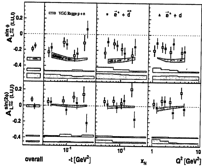
Рис. 7: Сравнение амплитуды асимметрий A_{L\to R}^{\sin\phi} и A_{LU}^1 .
