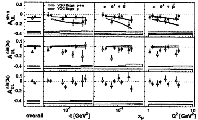
Рис. 8: Амплитуды асимметрии A_{UL} на протоне и дейтроне.
